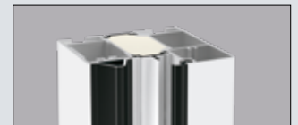
Thermisch getrennte Alu-Zarge A4
