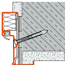
Diagonalbefestigung (Mauerwerk)
